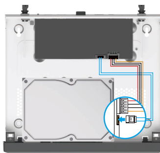
Adatkábeles csatlakozás
