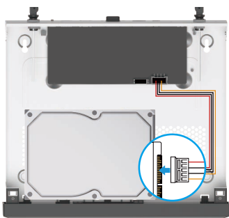
Tápkábel csatlakozás
